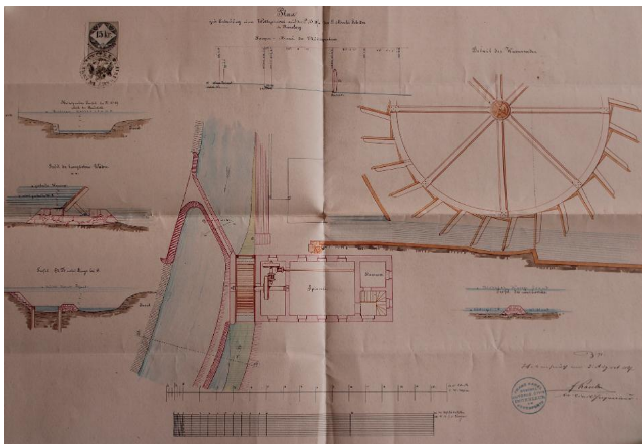
Plán přádelny z roku 1867: Soka Český Krumlov, fond Okresní úřad Vyšší Brod, Ú-71, sign. 9 20/54, karton 3.
